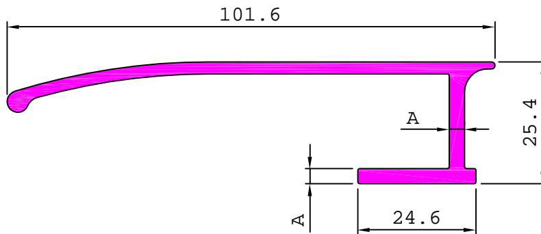
18555 0.686 kg/m
