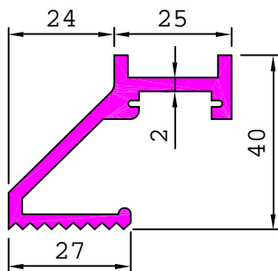
18555 0.686 kg/m
