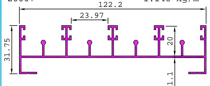
20667 1.148 kg/m
