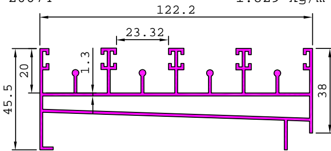
20674 1.829 kg/m
