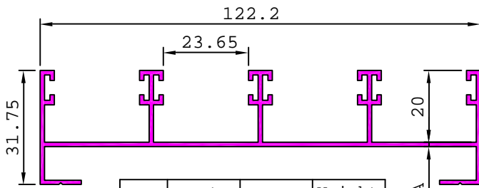
20833 1.398 kg/m
