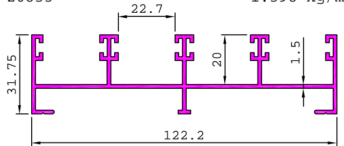
20833 1.398 kg/m
